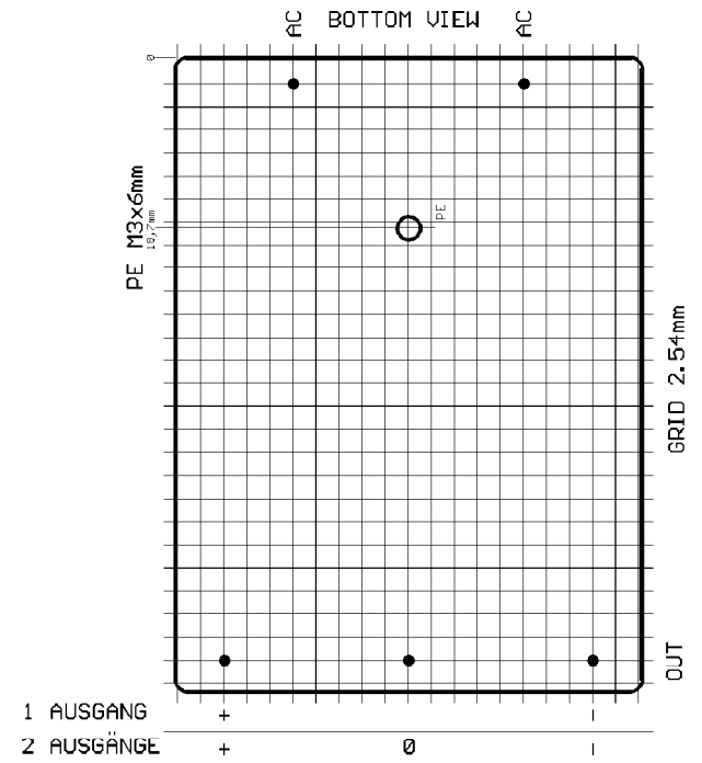
ANSCHLUSSBILD C BOTTOM VIEW
